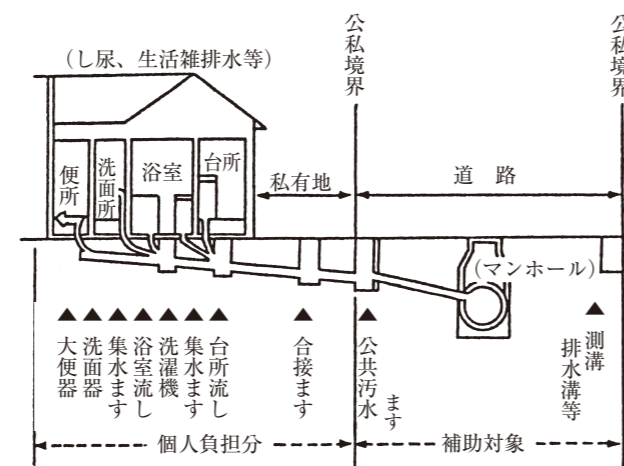
図2 一般住宅配管標準図
