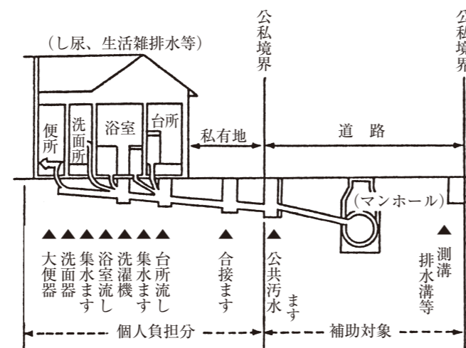
図2 一般住宅配管標準図
