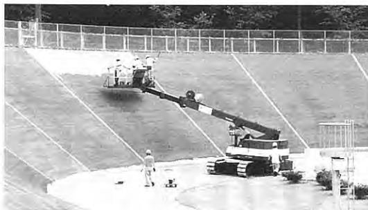
クレーンを使った補修工事
