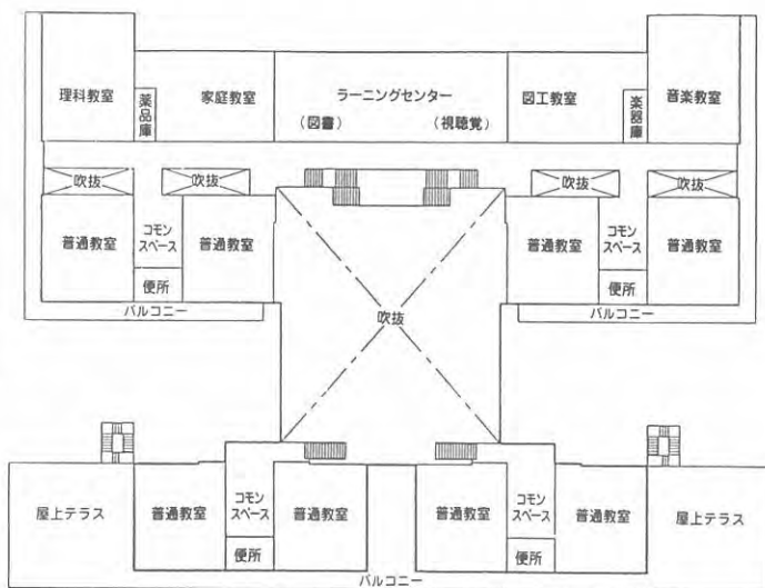
2階平面図
