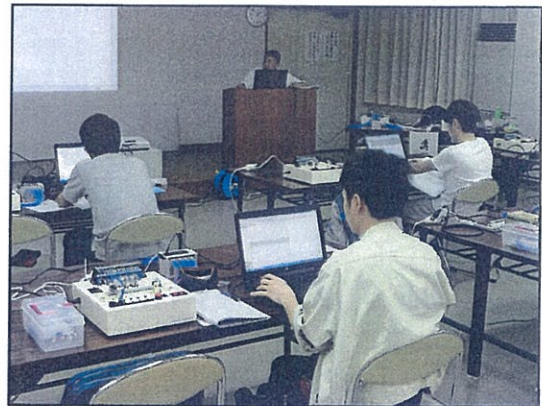
【シーケンス制御】
