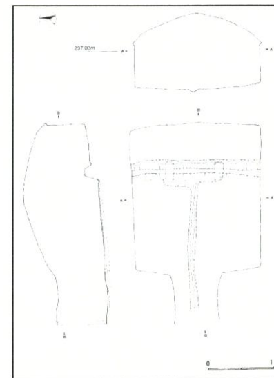
泉崎横穴の平面図
