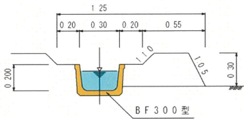
標準断面図（小用水路）
