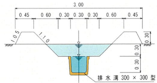
標準断面図（小排水路）
